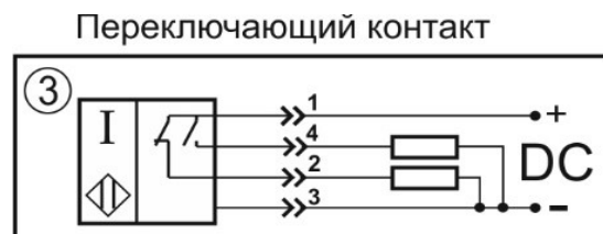
Схема соединения
