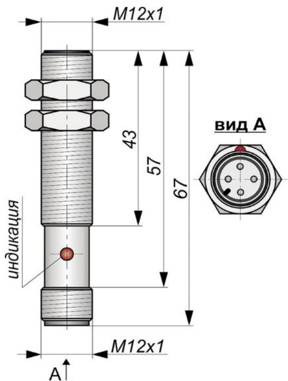
Габаритный чертеж
