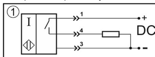
Цоколевка разъема
