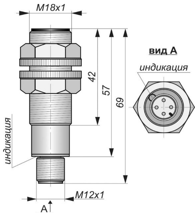
Габаритный чертеж
