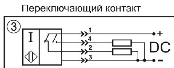
Цоколевка разъема
