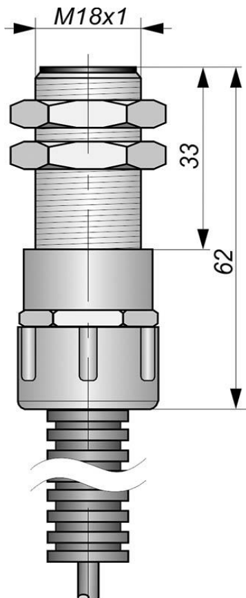
Габаритный чертеж
