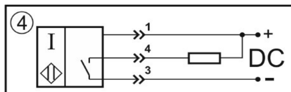
Цоколевка разъема
