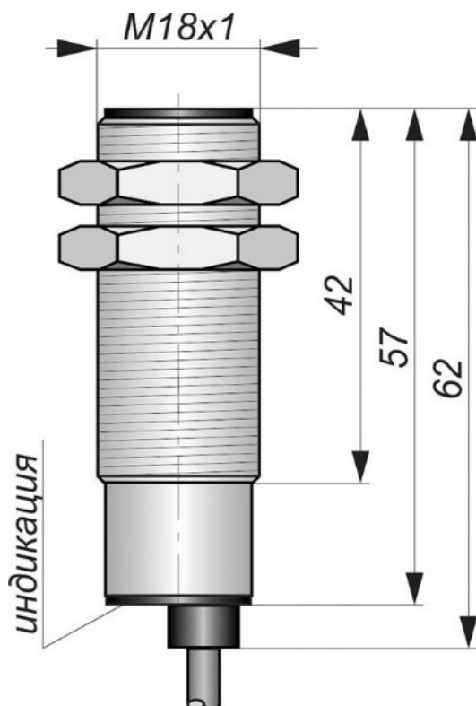
Габаритный чертеж
