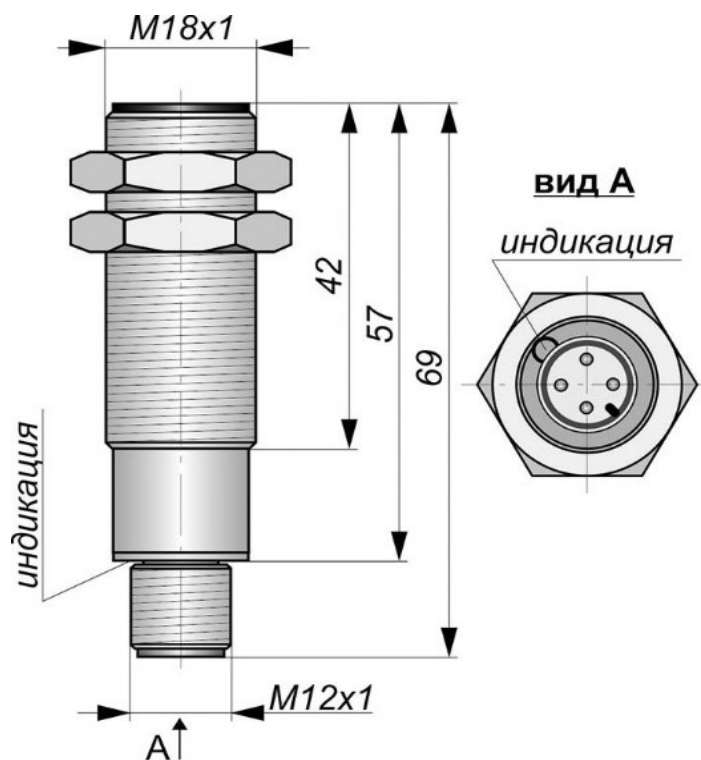
Габаритный чертеж
