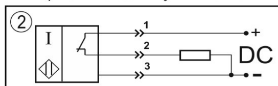
Цоколевка разъема
