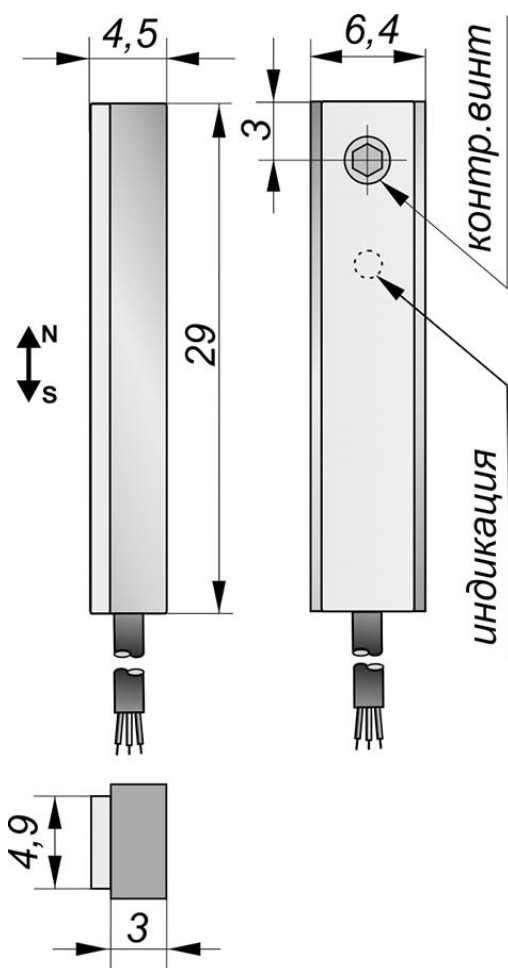
Габаритный чертеж
