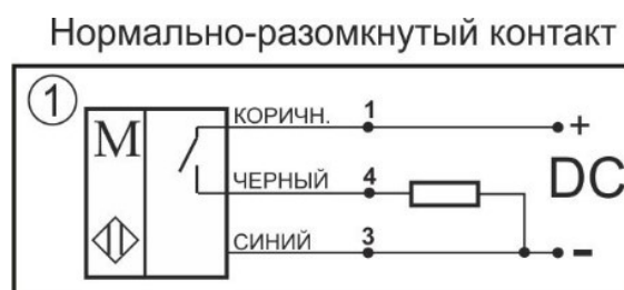
Схема соединения
