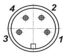
Цоколевка разъема
