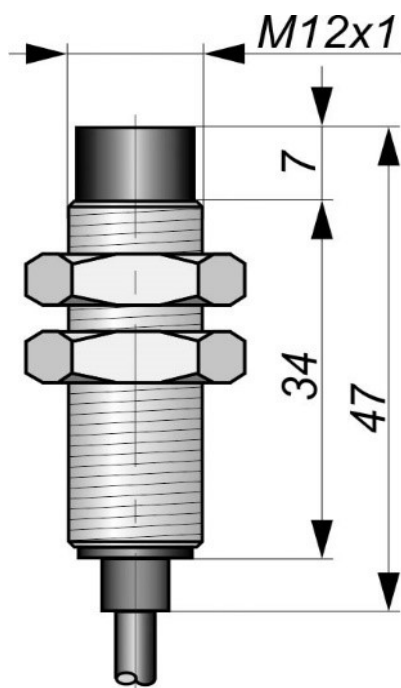
Габаритный чертеж
