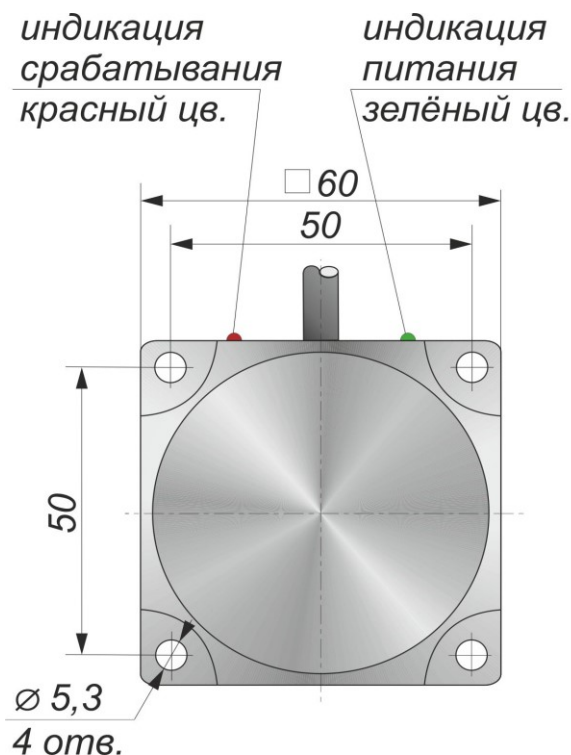
Габаритный чертеж
