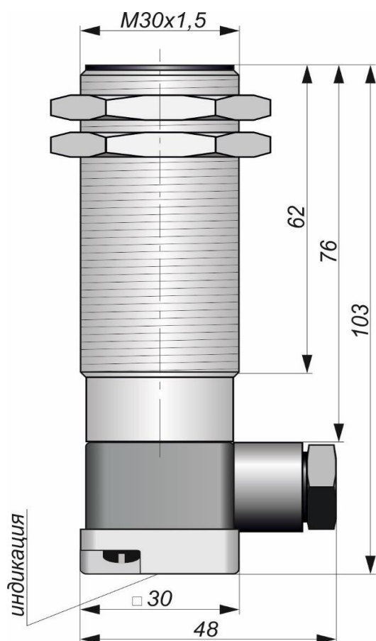
Габаритный чертеж
