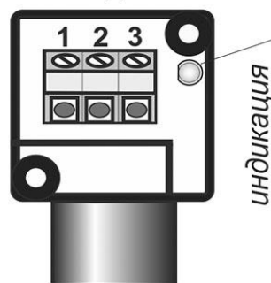
Цоколевка клеммной колодки
