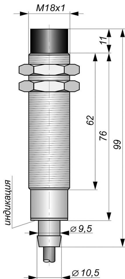
Габаритный чертеж
