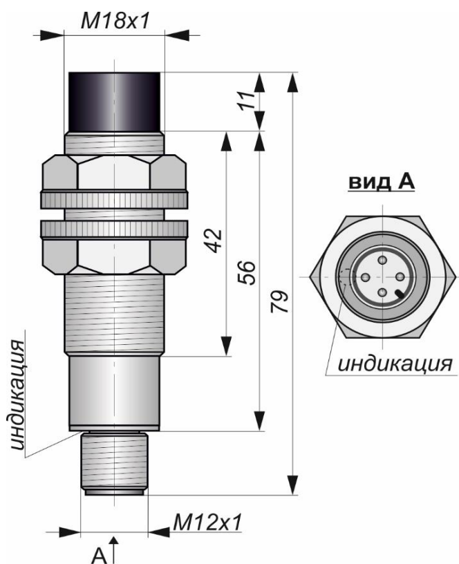
Габаритный чертеж
