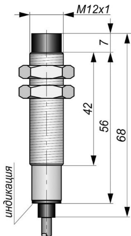
Габаритный чертеж
