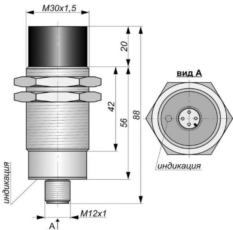
Габаритный чертеж
