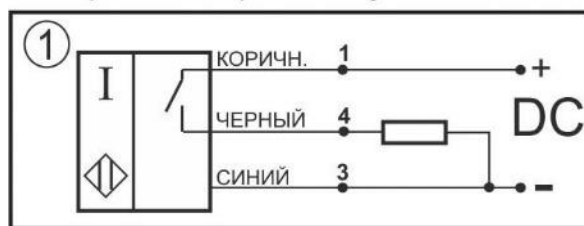
Нормально-разомкнутый контакт
