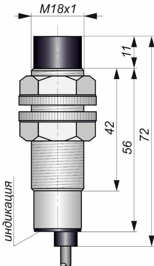
Габаритный чертеж
