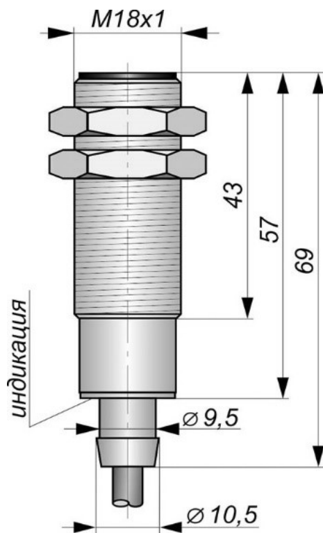
Габаритный чертеж
