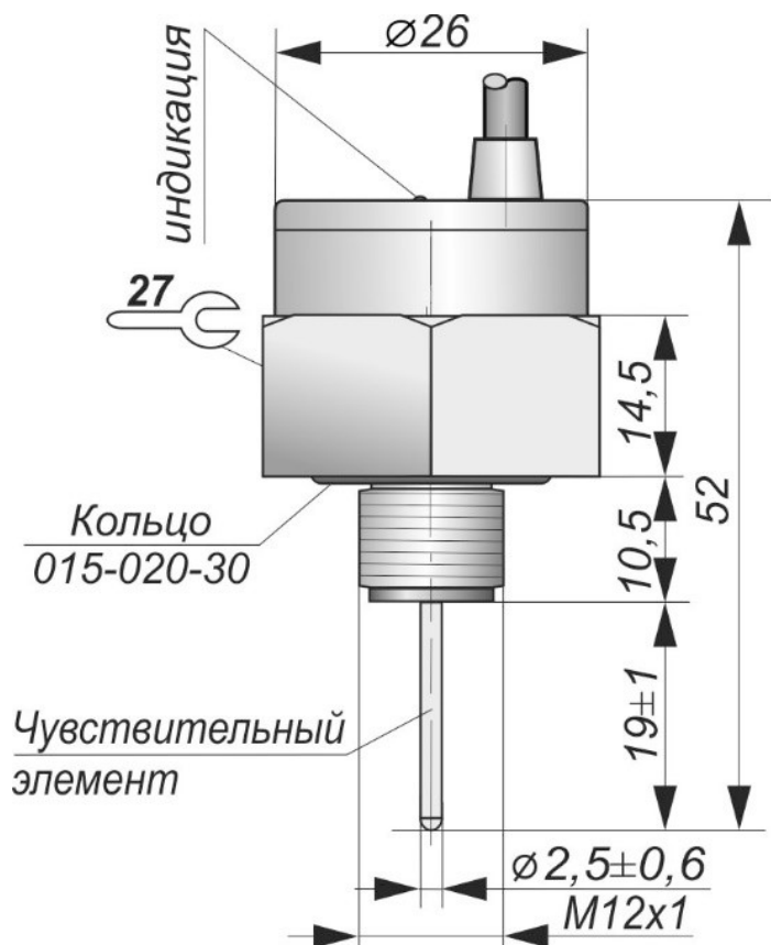
Габаритный чертеж
