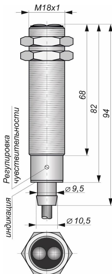
Габаритный чертеж
