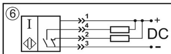
Переключающий контакт
