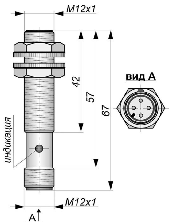
Габаритный чертеж
