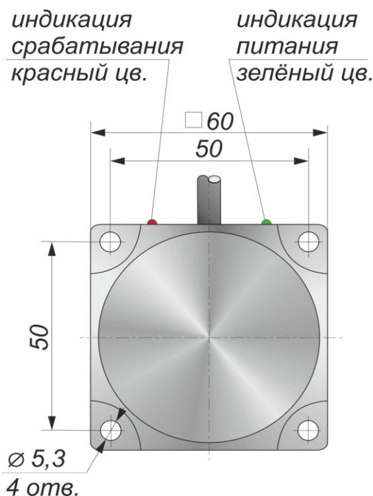
Габаритный чертеж
