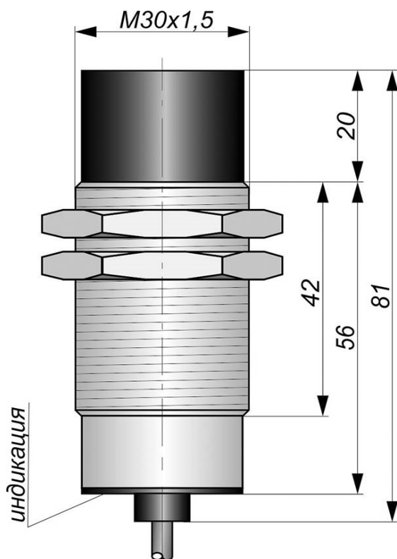
Габаритный чертеж
