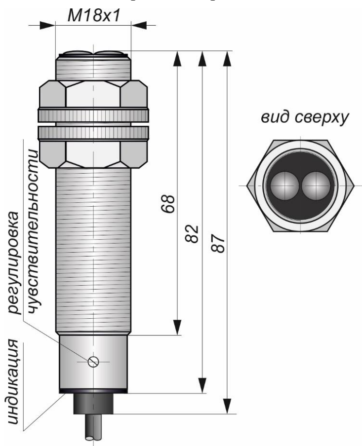
Габаритный чертеж
