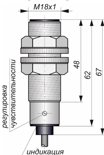
Габаритный чертеж
