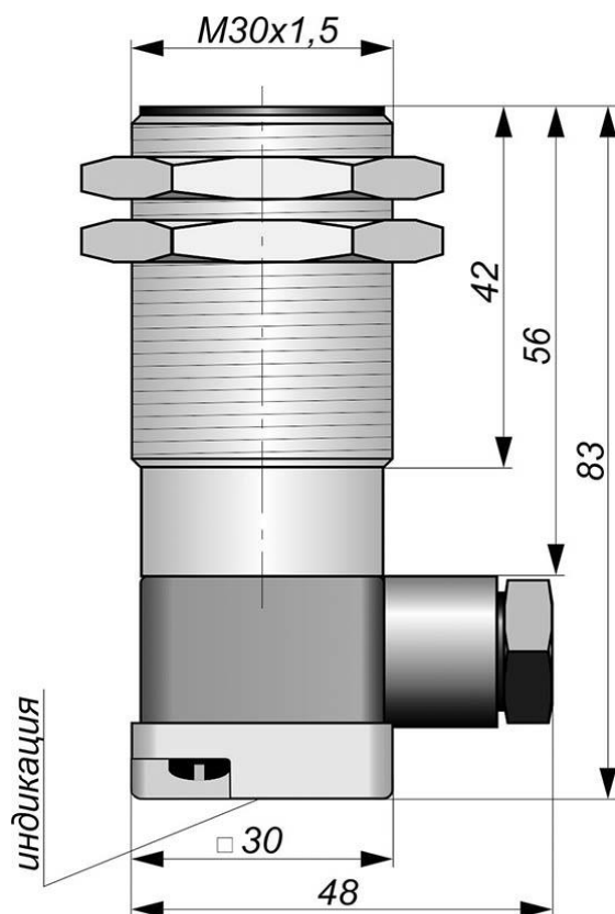
Габаритный чертеж
