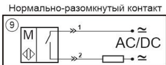
Схема соединения
