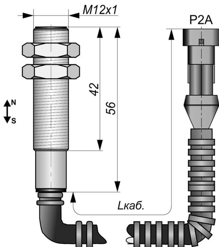
Габаритный чертеж
