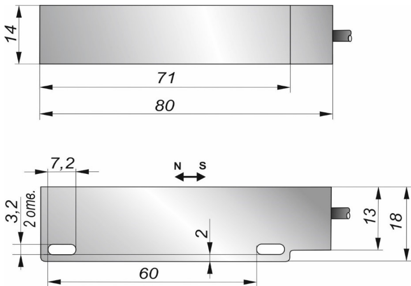
Габаритный чертеж
