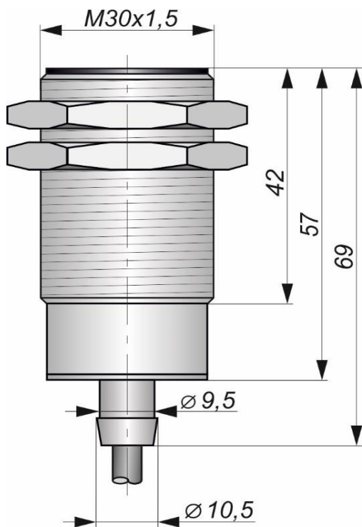
Габаритный чертеж
