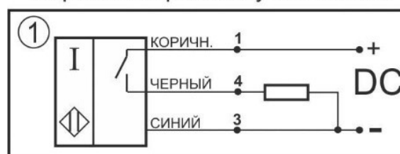
Схема соединения
