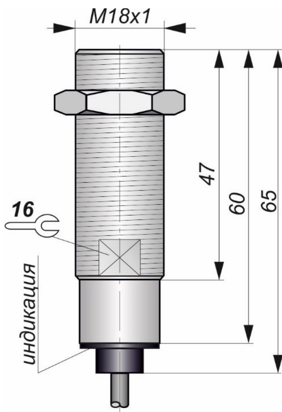
Габаритный чертеж
