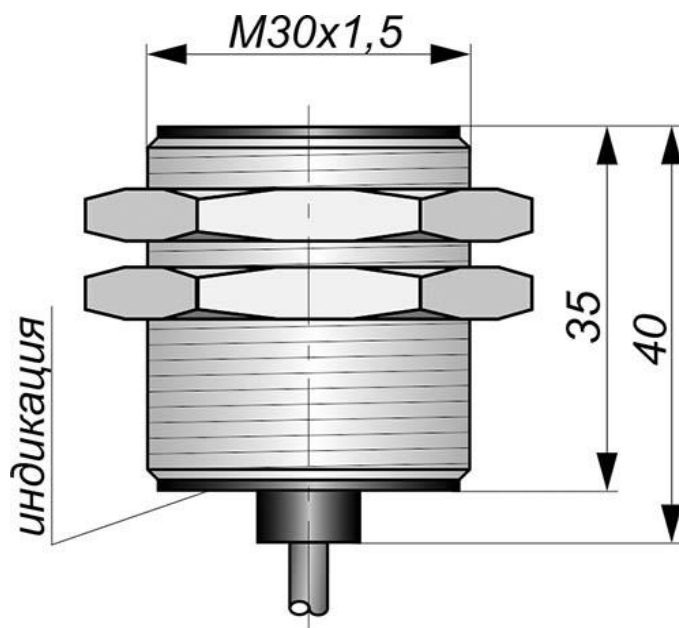
Габаритный чертеж
