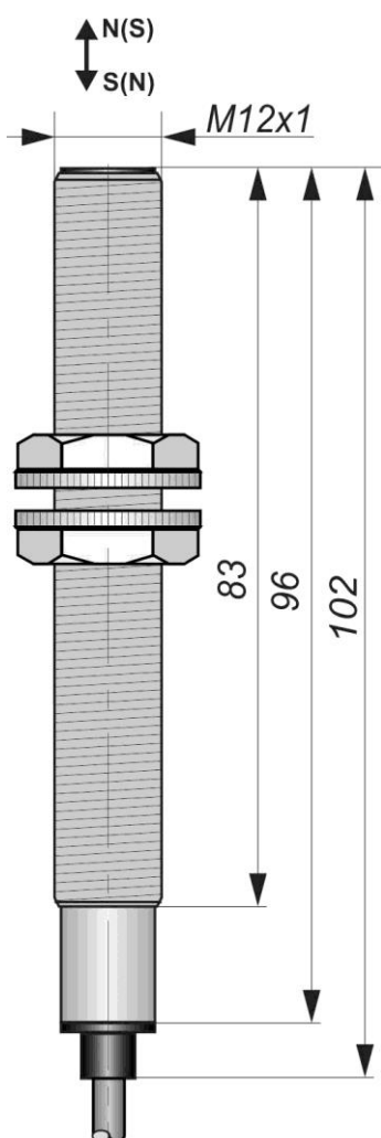
Габаритный чертеж
