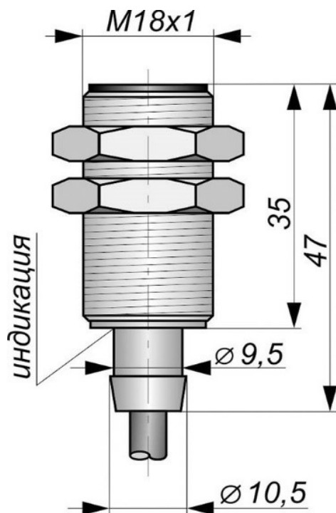
Габаритный чертеж
