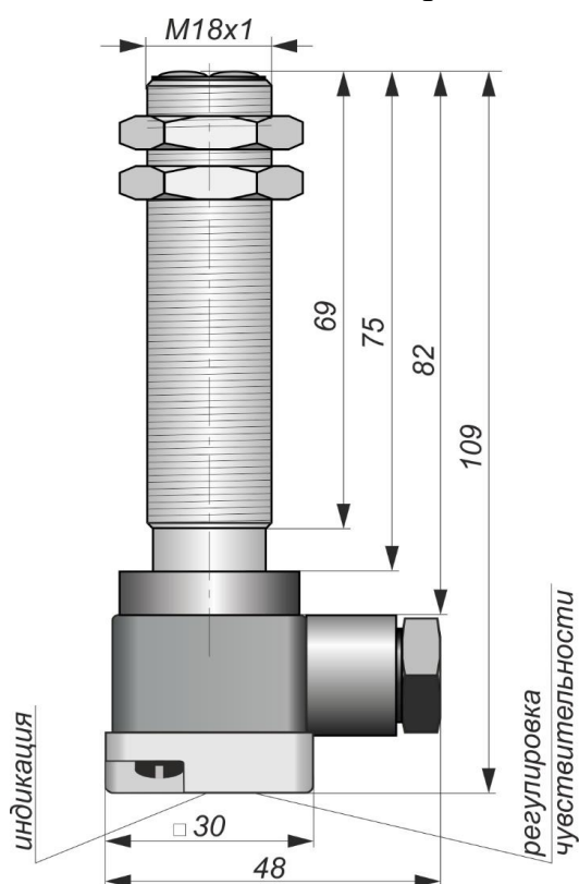
Габаритный чертеж
