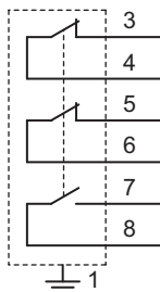
Рис. 7.4: Назначение контактов 8-полюсного штекерного разъема M12, ERS200-xxx-M12-xxx)
