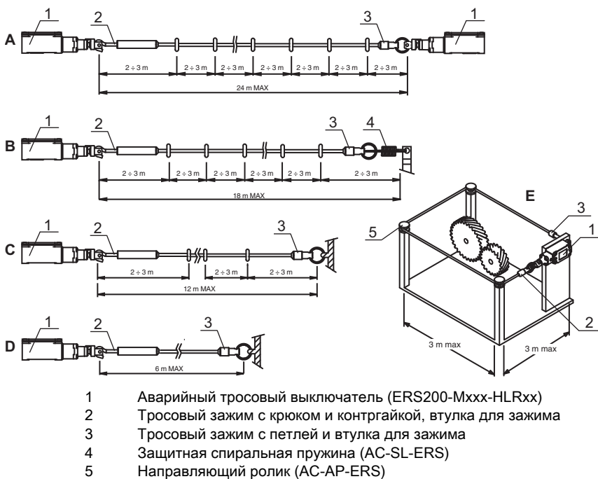
Рис. 6.1: Пример монтажа А–Е
