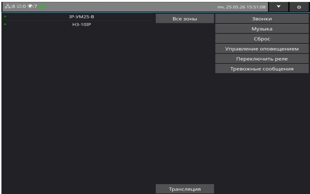
Рисунок 5 - Главная страница
