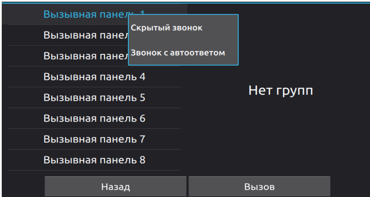
Рисунок 17 - Вид звонка
