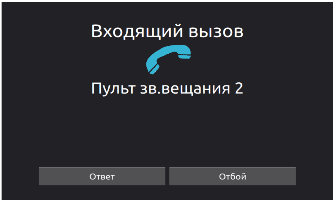
Рисунок 14 - Входящий вызов
