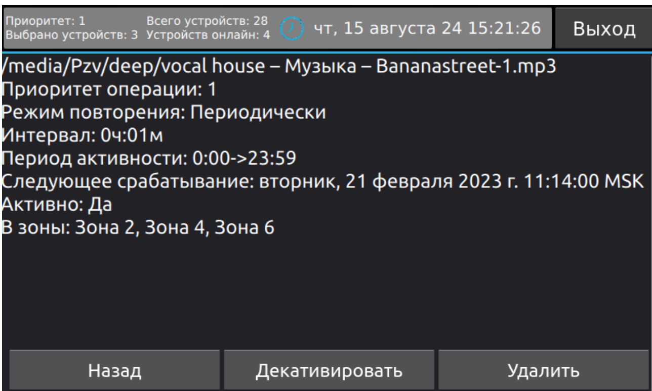
Рисунок 54 - Свойства расписания
