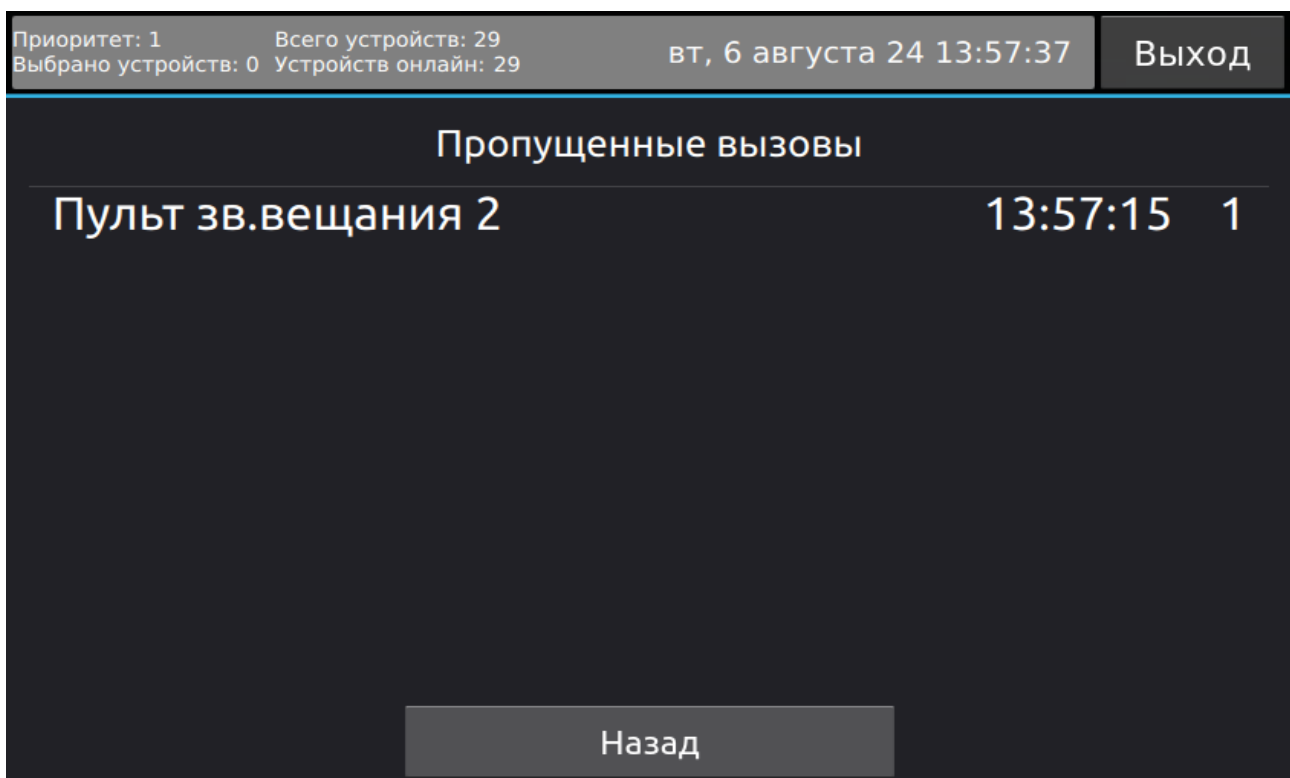
Рисунок 15 - Пропущенный вызов
