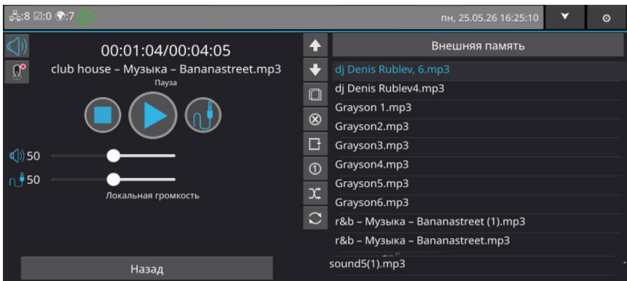
Рисунок 43 - Раздел «Музыка»
