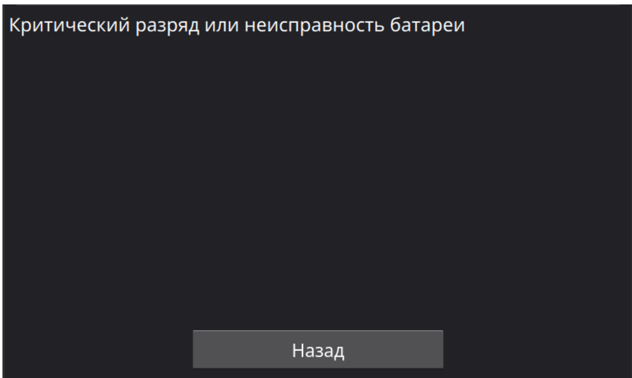
Рисунок 57 - Раздел «Неисправности»
