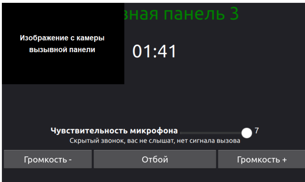
Рисунок 18 - Скрытый звонок
