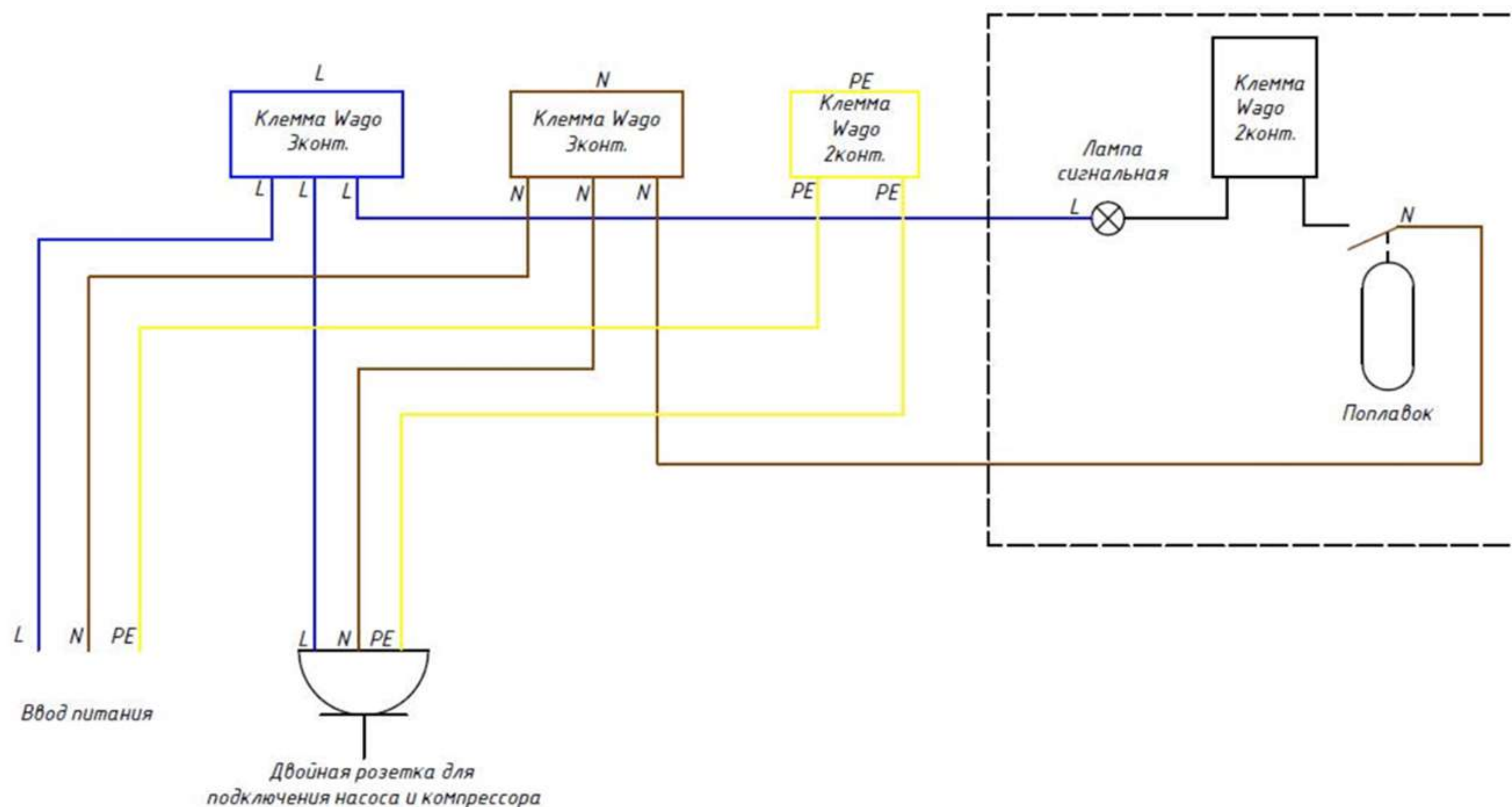
Схема подключений с аварийной сигнализацией
