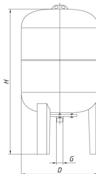
BASE 50 - 150 VERT
