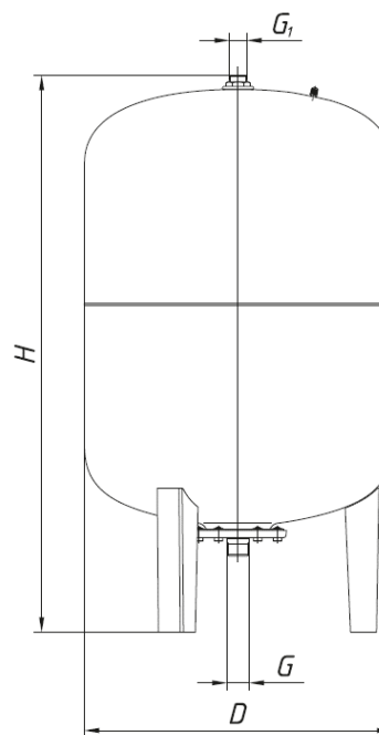
SIMPLE 80-150 VERT
