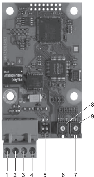
1-сұр. CIM 150 Profibus модулі
