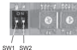
Նկար 6 Համաձայնեցնող ռեզիստորների միացնելն ու անջատելը
