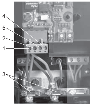
Նկար 3 Միացում ցանցին
