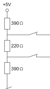
Նկար 5 Ներքին համաձայնեցնող ռեզիստորները
