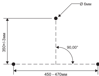
горизонтальное расположение
