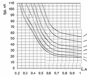
б) ШНП-1-10хВ, две шины 10 мм
