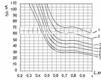
в) ШНП-2-10хВ, одна шина 10 мм
