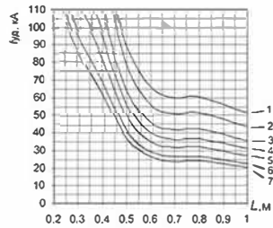
а) ШНП-1-10хВ, одна шина 10 мм
