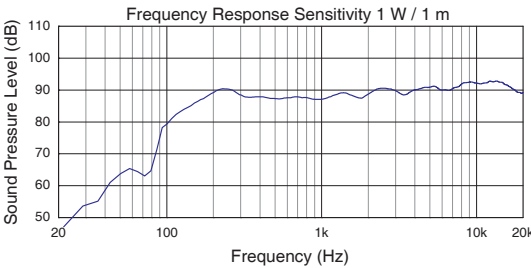
Graph 2# VLS 15 (EN 54)
