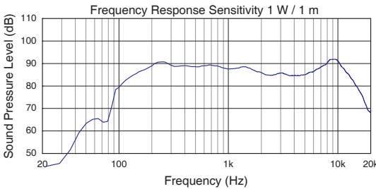
Graph 1# VLS 7 (EN 54)
