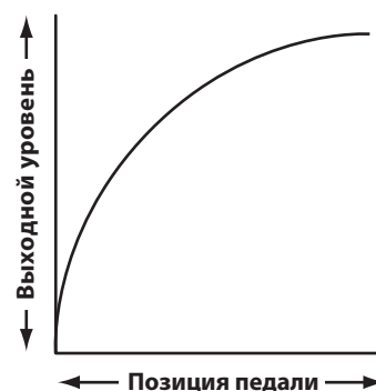
Кривая Fast
