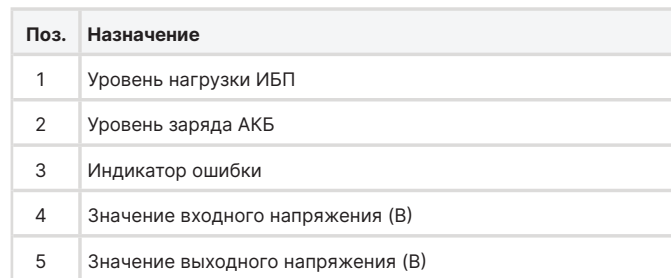
Рис. 6 Элементы индикации инвертора
