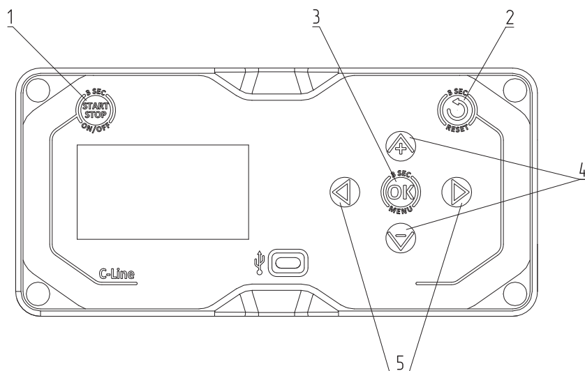
Рис. 5 Функциональные клавиши контроллера C-Line
