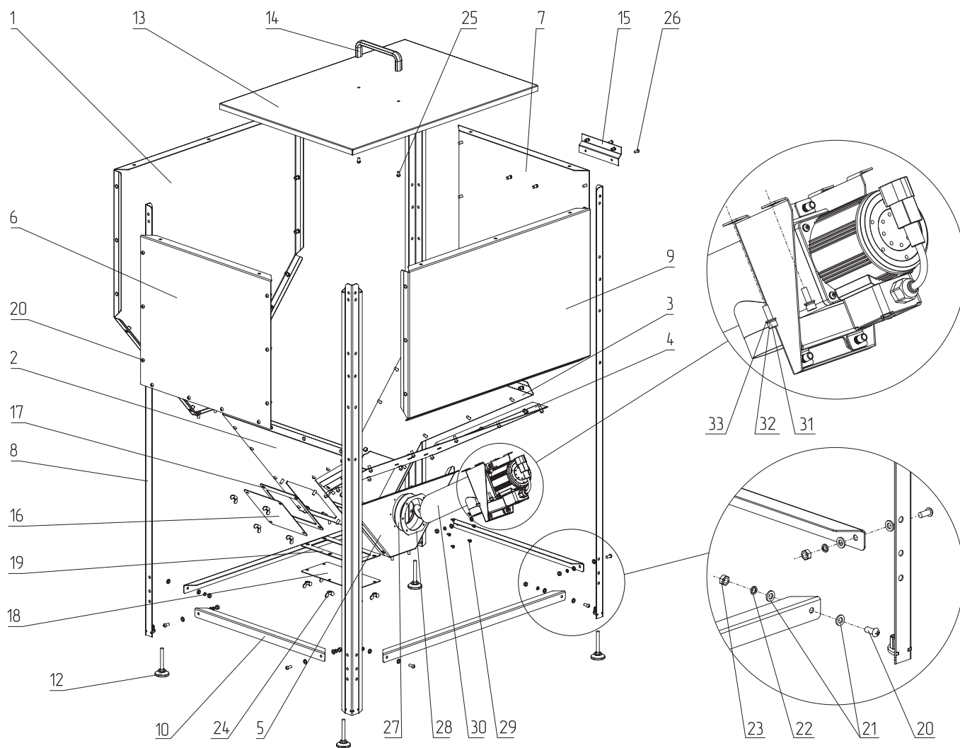
Рис. 4 Конструкция бункера
