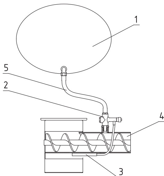
Рис. 6 Система охлаждения топливопровода
