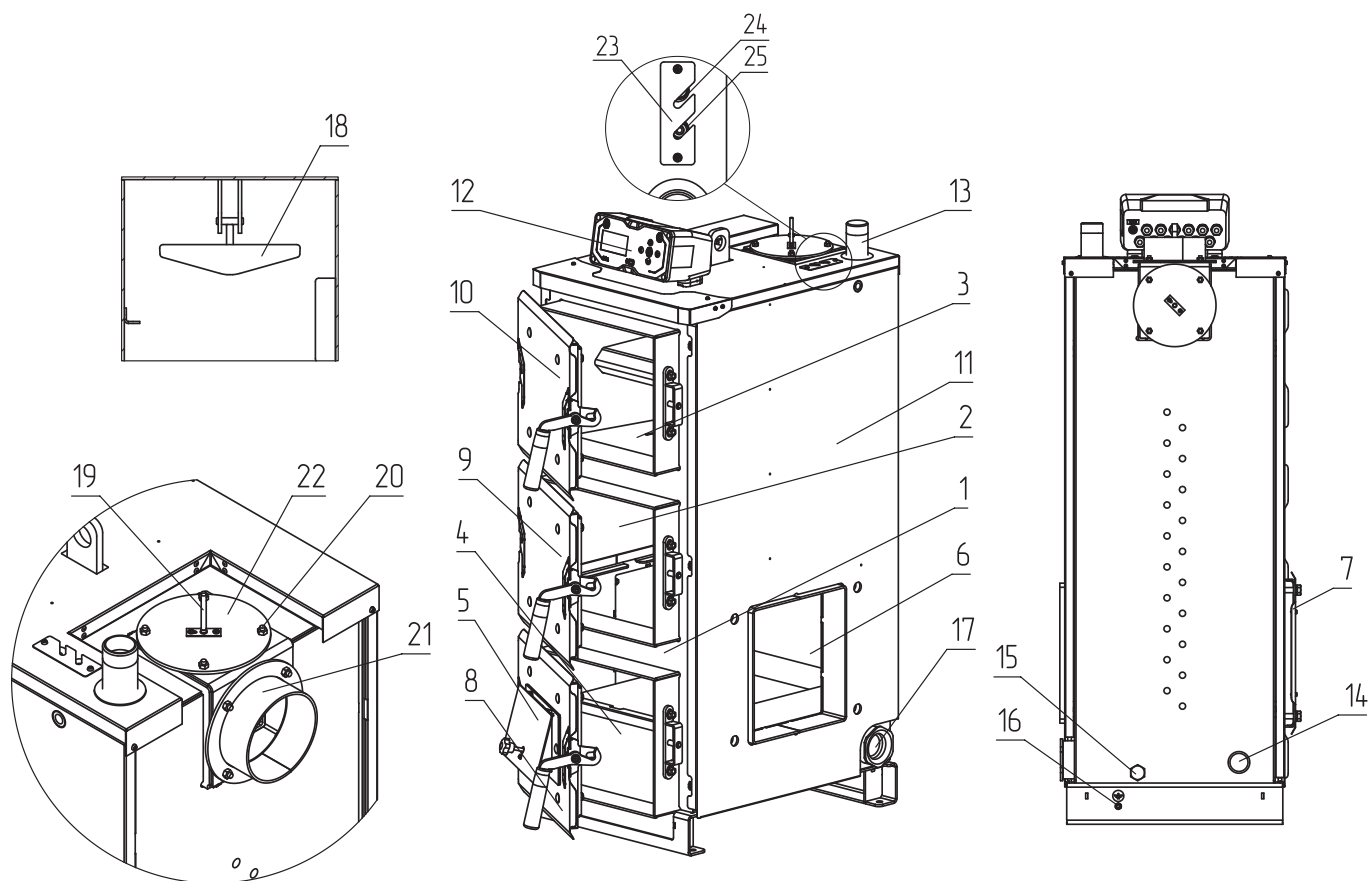
Рис. 2 Конструкция теплообменника котла ZOTA Focus
