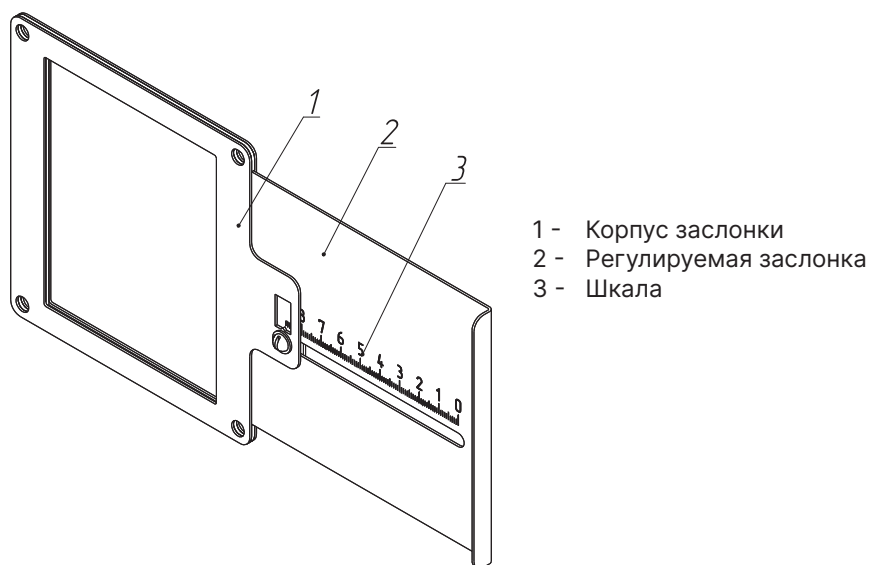
Рис. 15 Заслонка вентилятора
