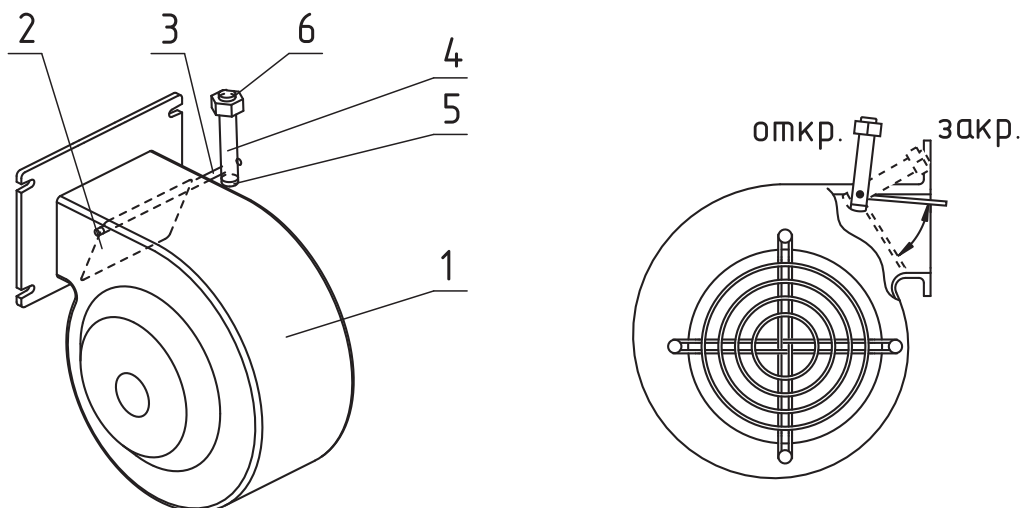
Рис. 7 Вентилятор наддува
