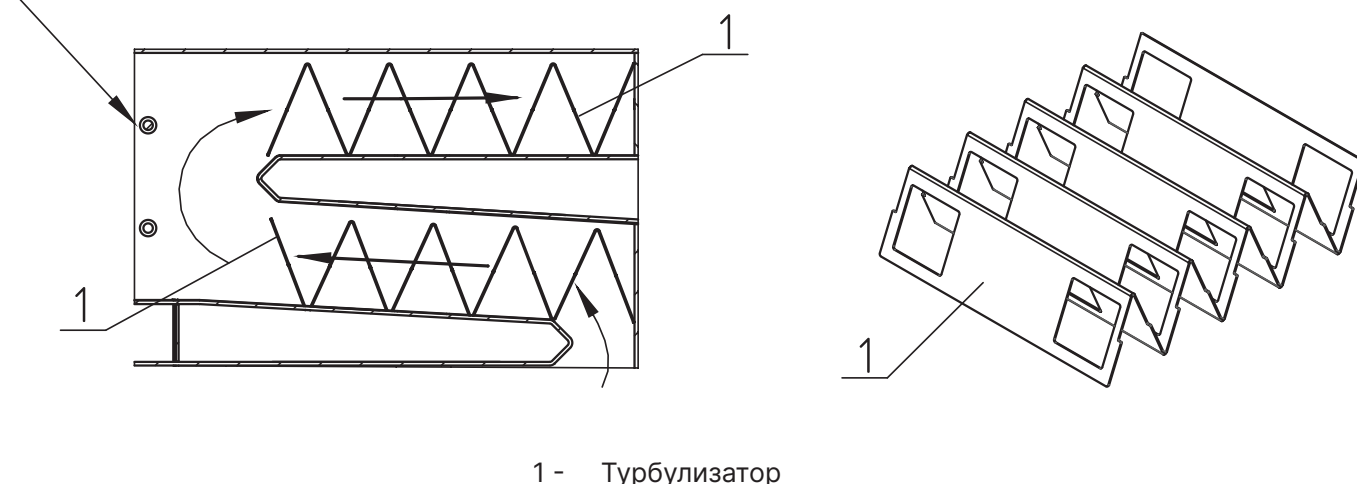
Рис.10 Установка турбулизаторов
