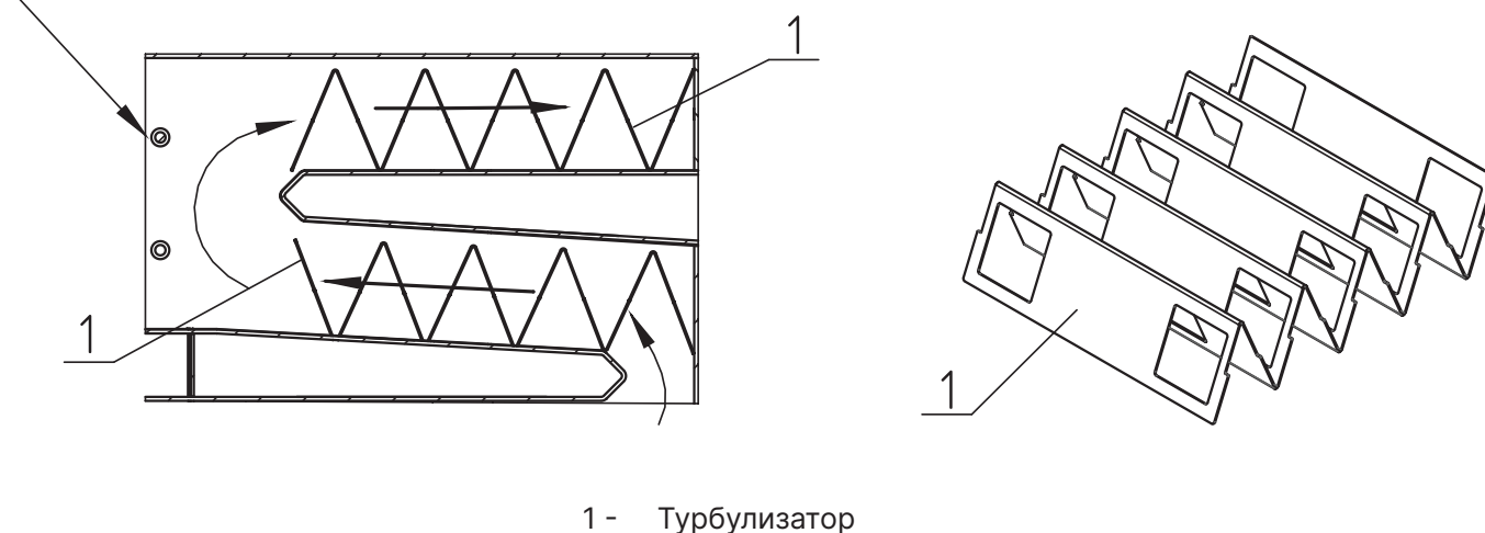
Рис.10 Установка турбулизаторов
