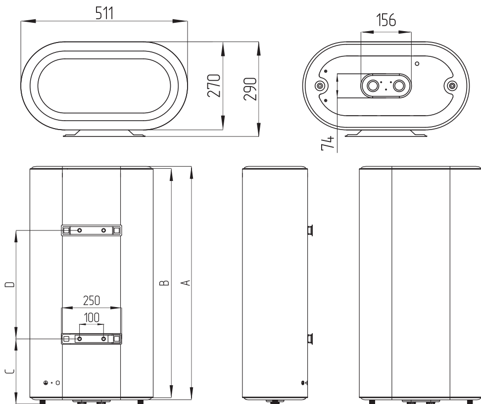
Рис. 3 Габаритные размеры водонагревателя ZOTA NELMA
