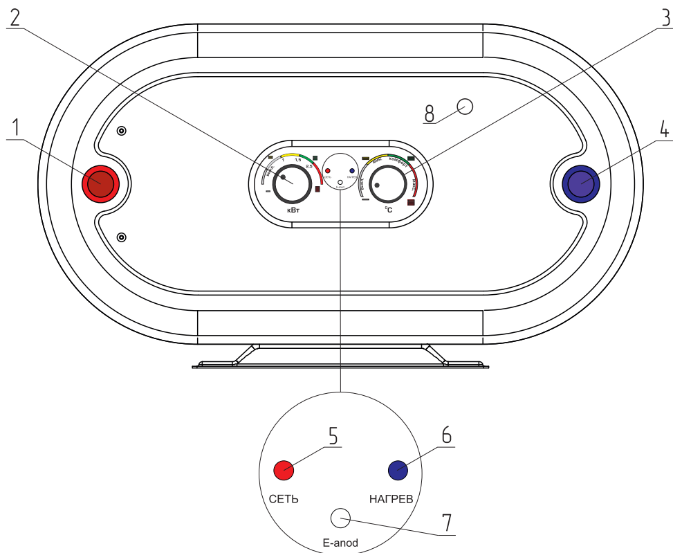
Рис. 1 Устройство водонагревателя ZOTA NELMA
