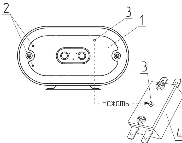
Рис. 5 Термовыключатель
