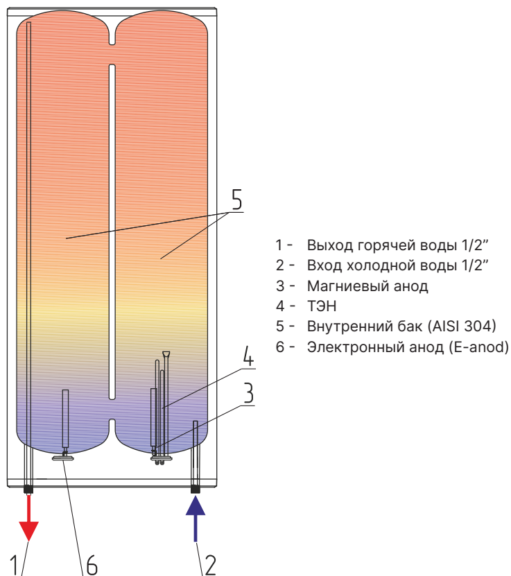
Рис. 2 Внутреннее устройство водонагревателя
