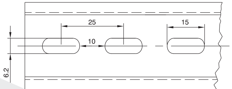
Рис.5 Размеры отверстий PM-35/15/П и PM-35/7,5/П
