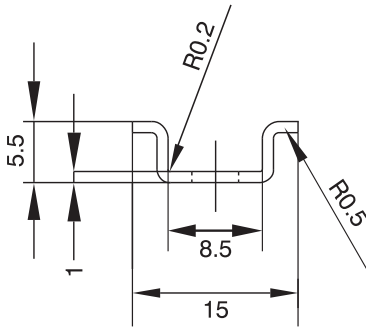
Рис.1 Размеры PM-15/5,5
