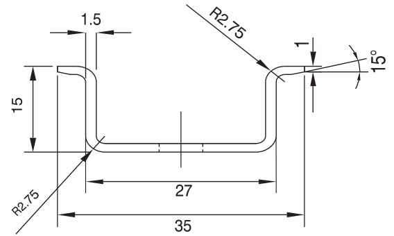
Рис.3 Размеры PM-35/15
